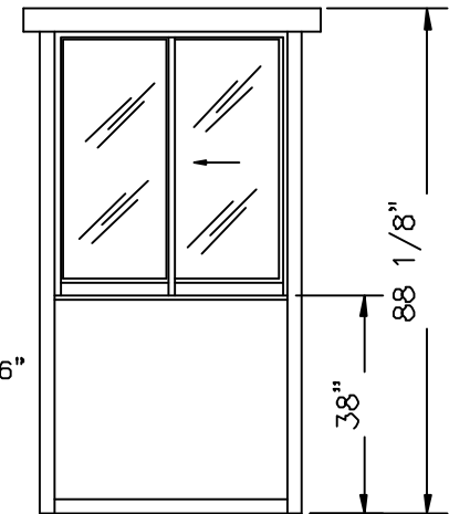
ELEVATION B
